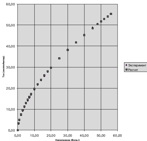
Вольтамперная характеристика лампочки накаливания
