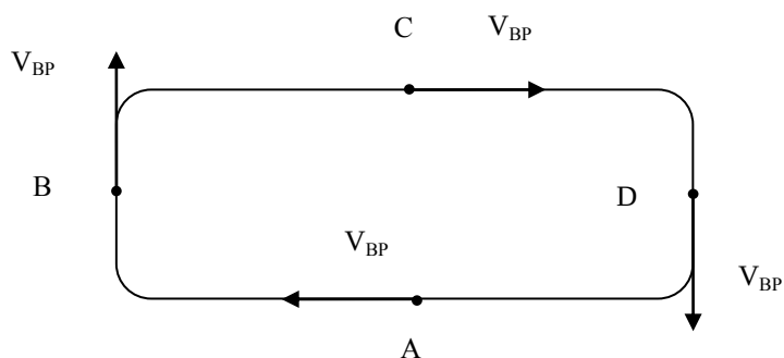
Система отсчета S («кабина вездехода»)
